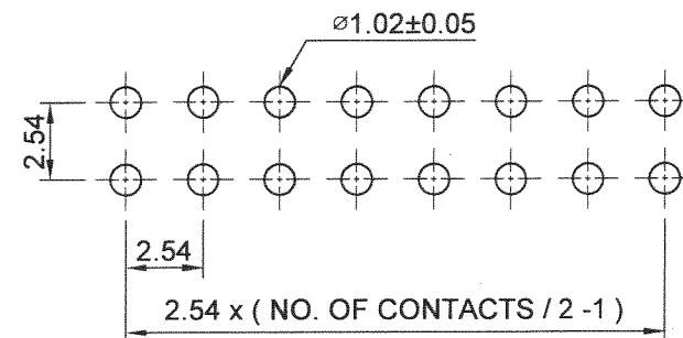
P.C.Board Layout
